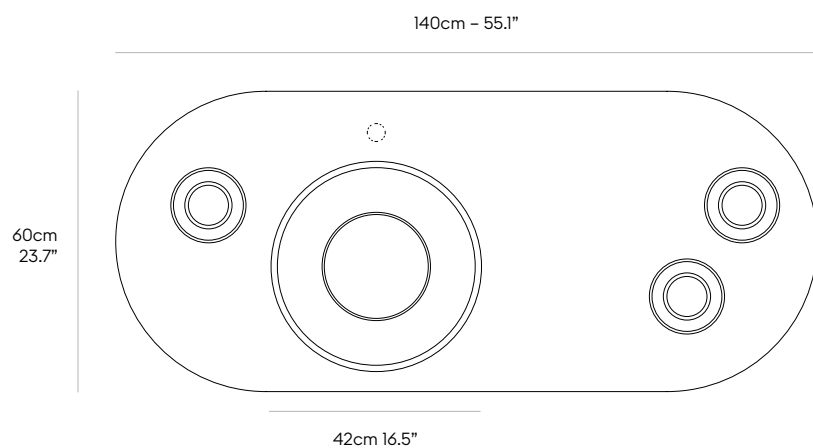
Product dimensions / Dimensioni del prodotto
